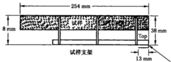
图 3 插在试样支架上的试样(侧组图)
