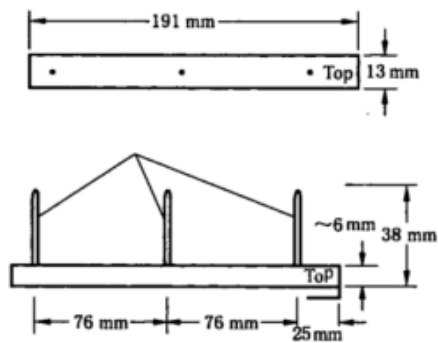
图 2 试样支架主要尺寸
